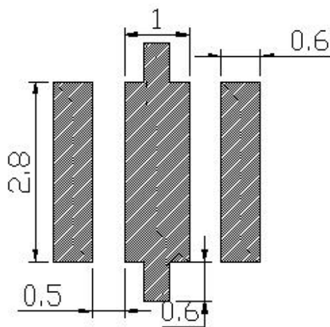
焊盘建议图
