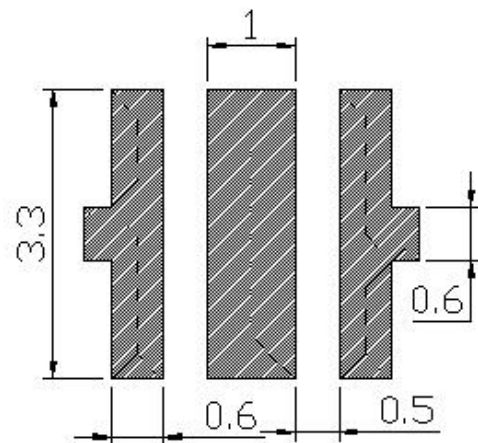
焊盘建议图
