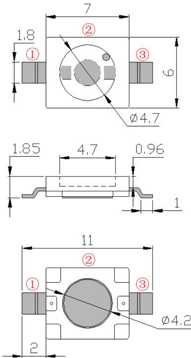
焊盘建议图
