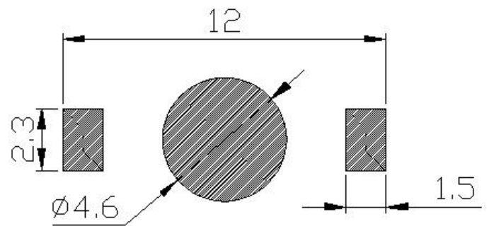
焊盘建议图
