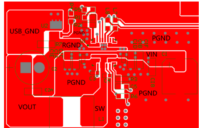
Top Layer
