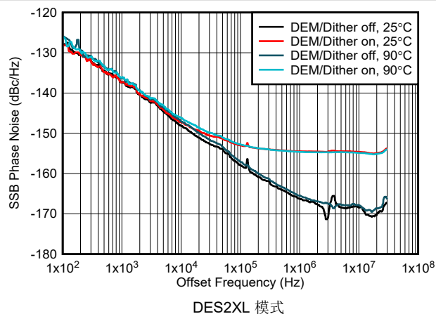
图 6-205. 1GHz 条件下相位噪声与偏移频率间的关系
