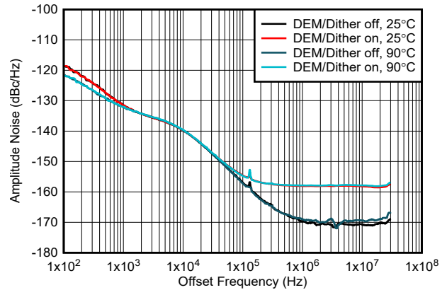
图 6-210. 1GHz 条件下振幅噪声与偏移频率和温度间的关系
