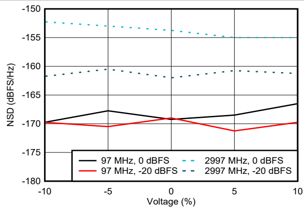
图 6-87. NSD 与电源电压间的关系
