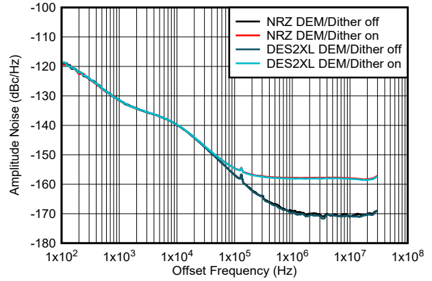
图 6-208. 1GHz 条件下振幅噪声与偏移频率间的关系
