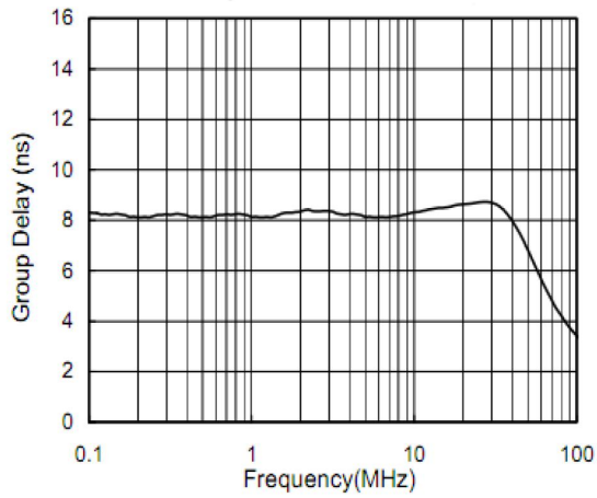
群延时与频率的关系
