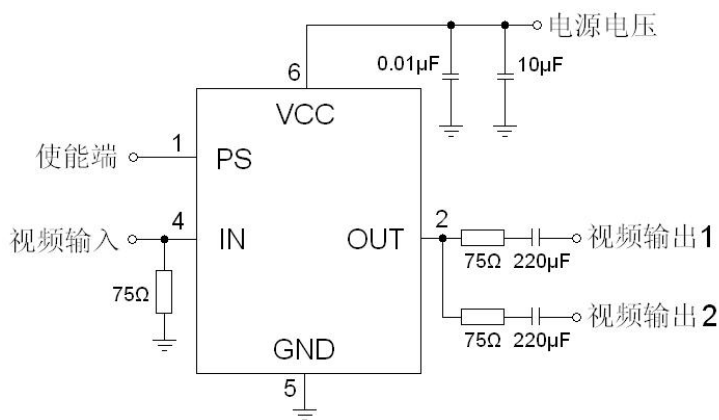
图 3 机顶盒中直流耦合电路原理图
