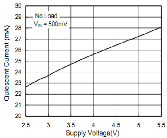
静态电流与电源电压的关系
