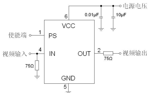
图 1 直流耦合应用原理图
