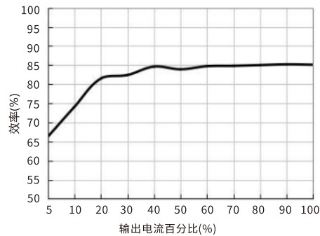
效率Vs输出负载(Vin=24V) URB2405YMD-6WR3
