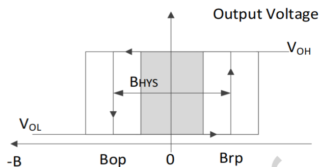
S0T23-3L输出状态
