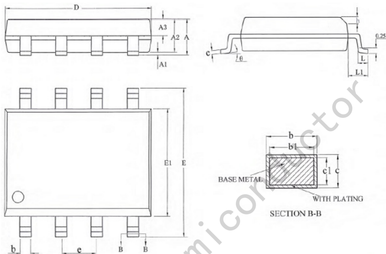
SOIC-8 Package Dimensions
