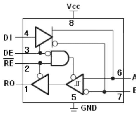
图2: SN75LBC184逻辑图
