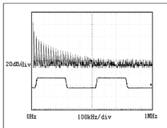
图 13: 传输 20kHz 信号时 SN75LBC184驱动器输出波形和 FFT 图
