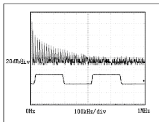
图 13: 传输 20kHz 信号时 SN65LBC184驱动器输出波形和 FFT 图
