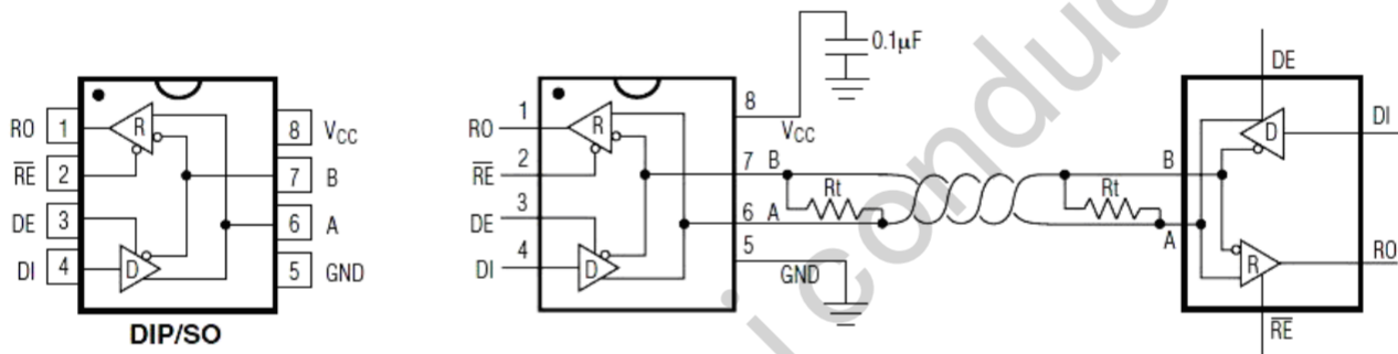
图 3: SN65LBC184典型半双工应用电路
