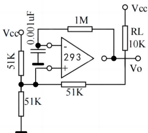
方波振荡器
