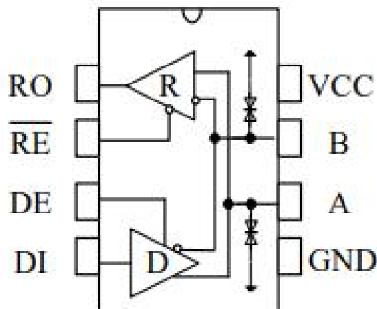
图 1 BL3085 (I47) 引脚分布图
