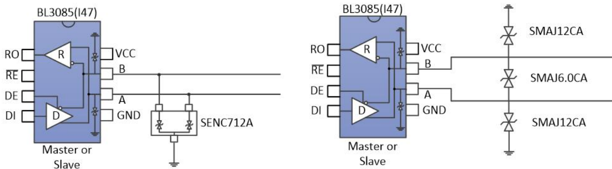
图 11 端口防护方案
