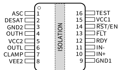
NSI6611ASC-DSWR
