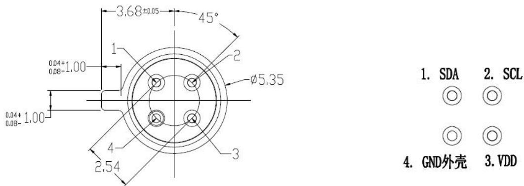
图 8. 基体底视图
