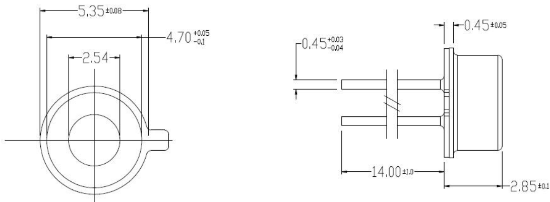
图 9. 基体轮廓尺寸
