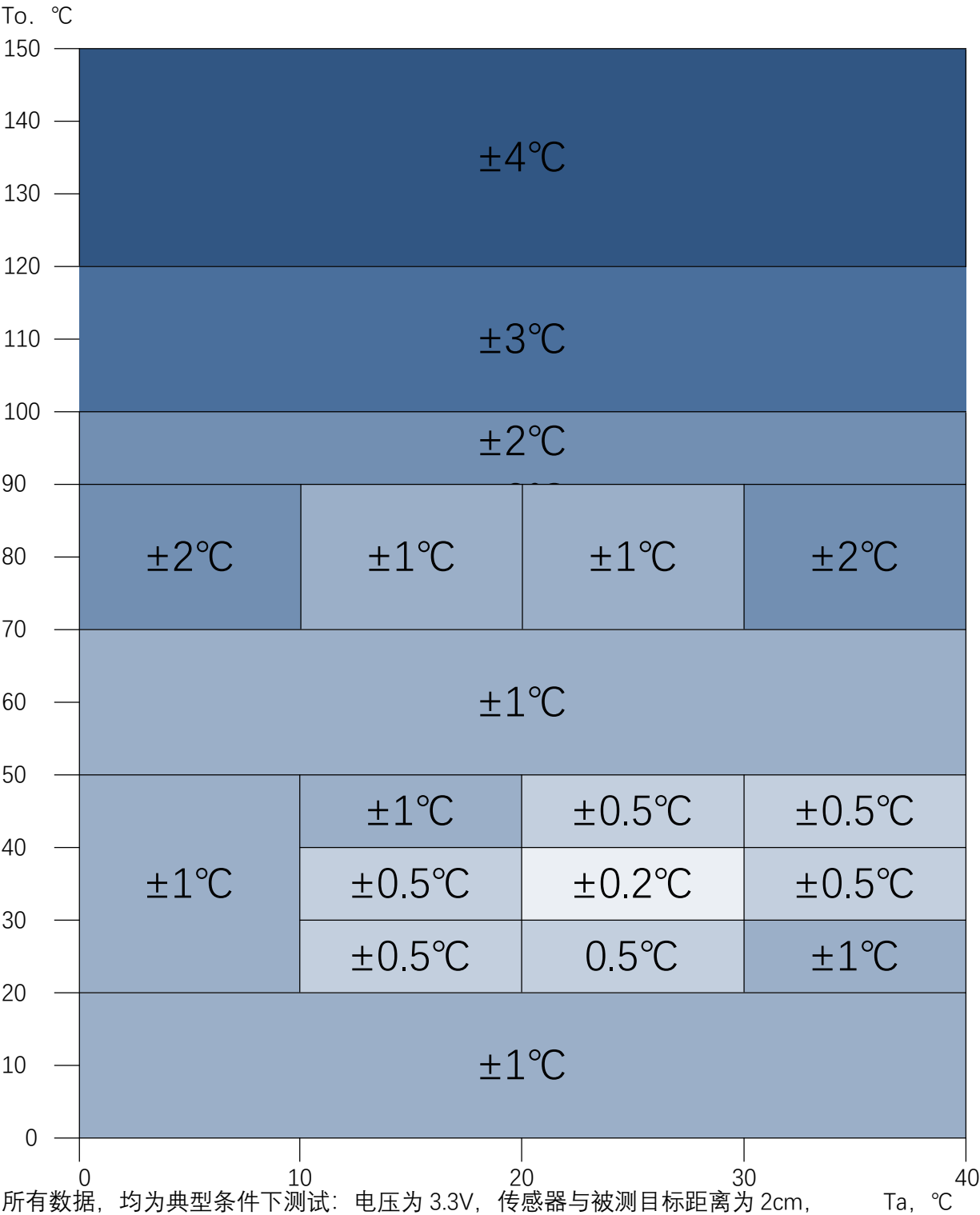
图 3.SL-W-TRS-5.5D (Ta,To) 的标准精度
