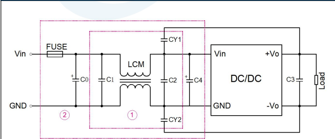
EMC 推荐电路（图 3）
