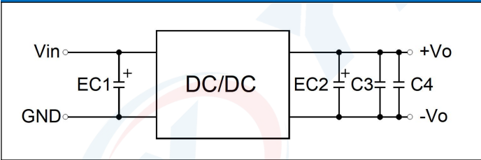
应用电路（图 2）
