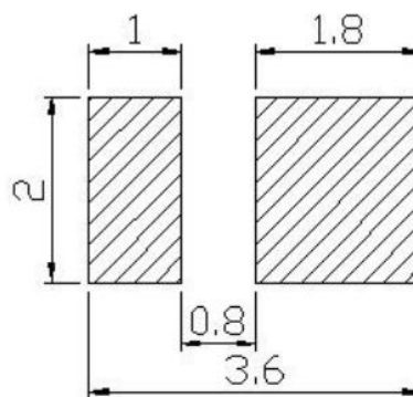
焊盘建议图
