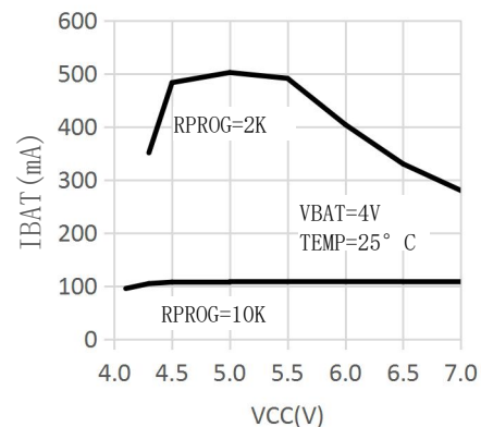
充电电流与电源电压的关系曲线
