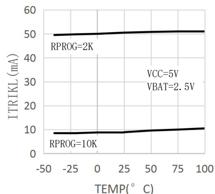
涓流充电电流与温度的关系曲线
