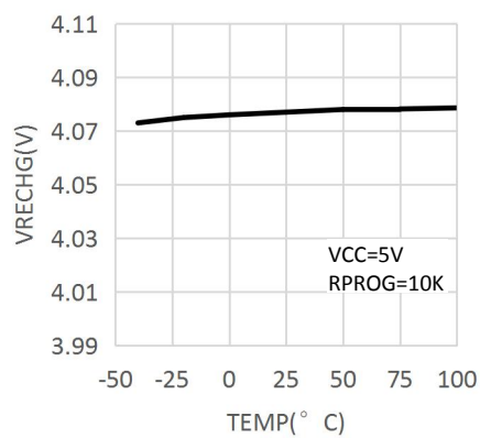
再充电电压门限与温度的 关系曲线
