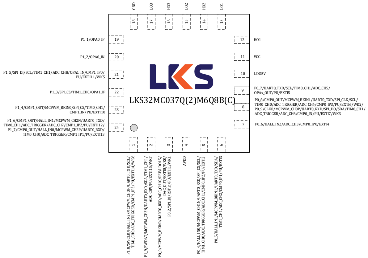
图 3-17 LKS32MC037Q(2)M6Q8B(C)管脚分布图
