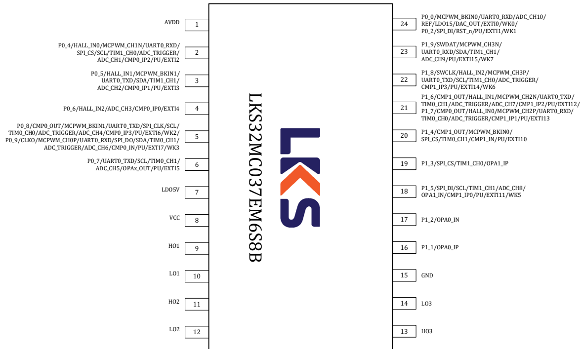
图 3-11 LKS32MC037EM6S8C 管脚分布图
