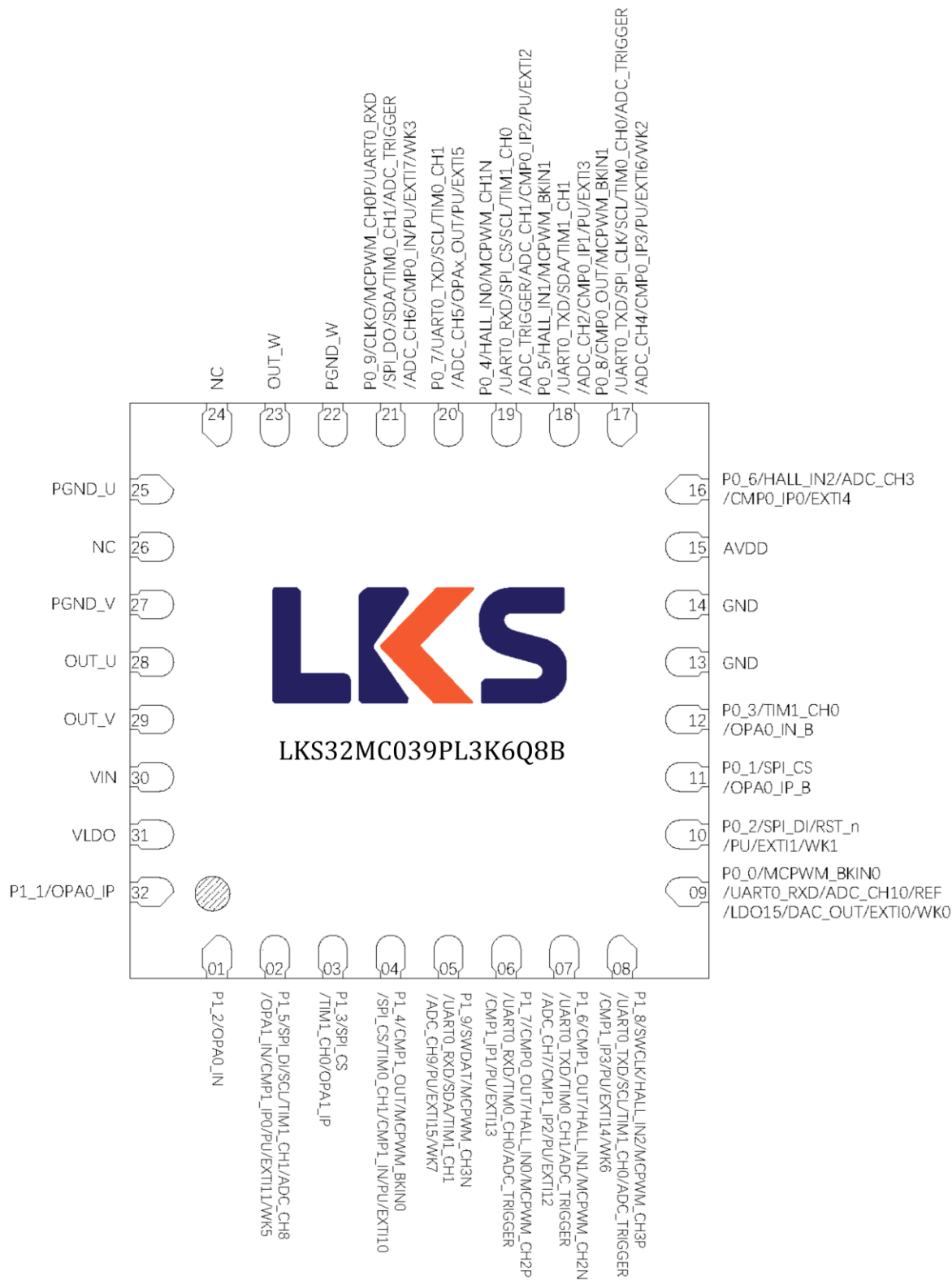
图 3-23 LKS32MC039PL3K6Q8B(C)管脚分布图
