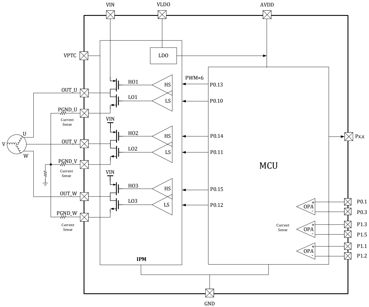
图 3-22 LKS32MC037QM6Q8 预驱连接示意图
