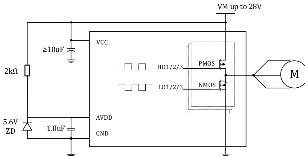
图 22-1 集成 P-N 功率 MOS 型 3P3N 栅极驱动模块典型应用图
