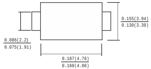
SMB(DO-214AA)
