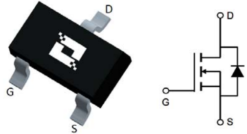
SOT23
