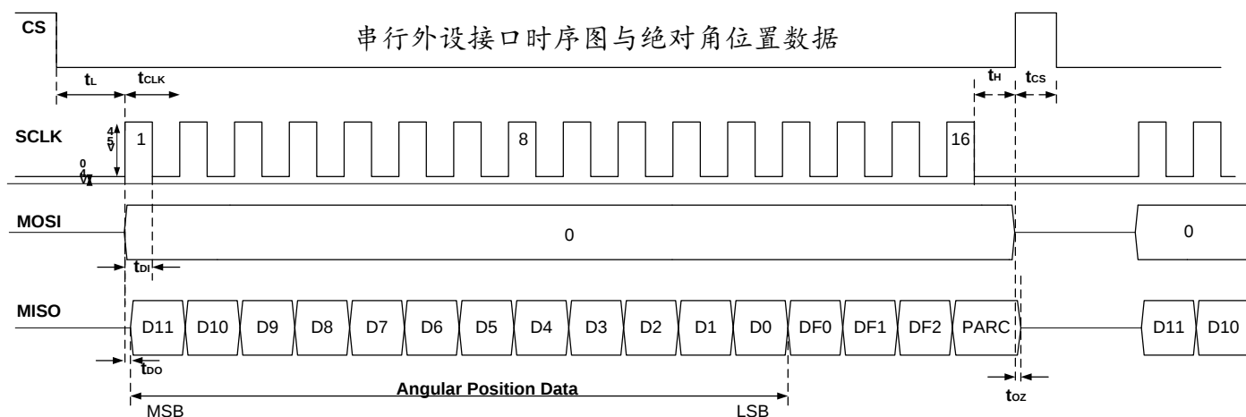
SPI 时序图
