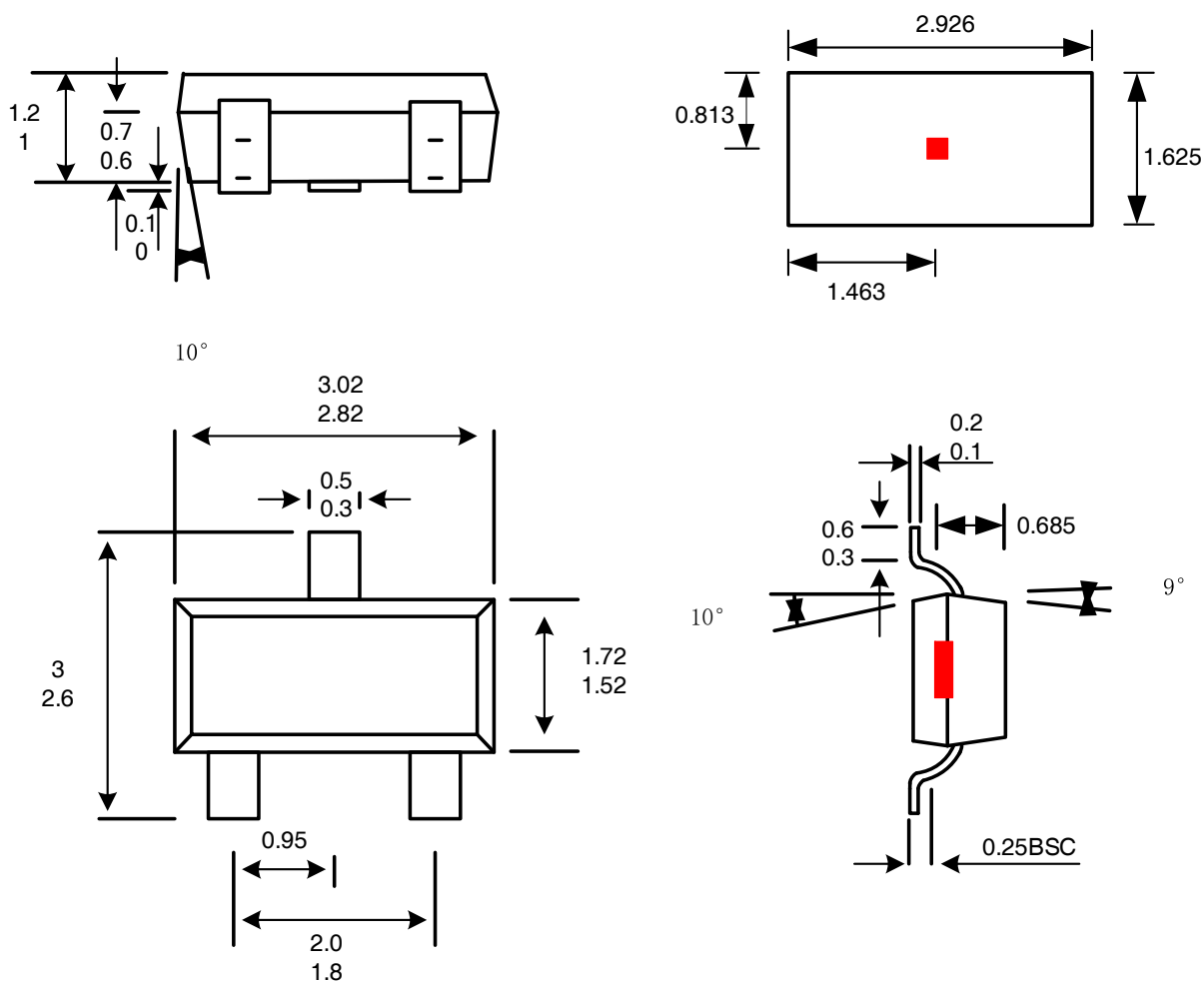
3-脚 SO封装
