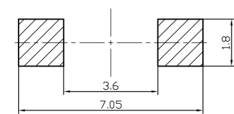
安装参考图
