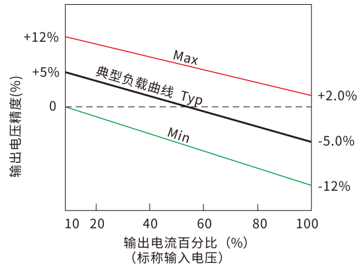
误差包络曲线图 3.3Vdc输出
