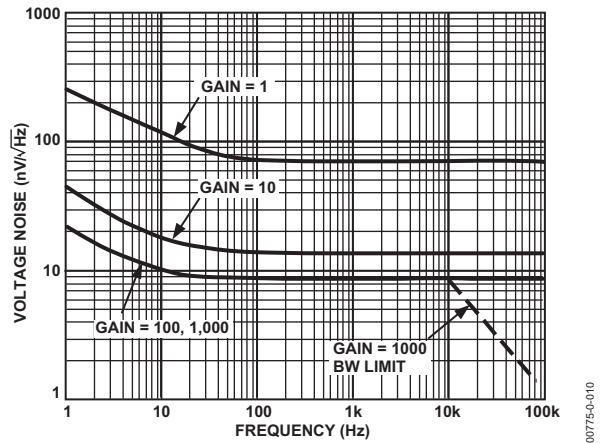
图10. 电压噪声谱密度与频率的关系 ( G = 1-1000 )
