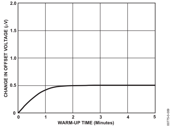
图9. 输入失调电压变化与预备时间的关系
