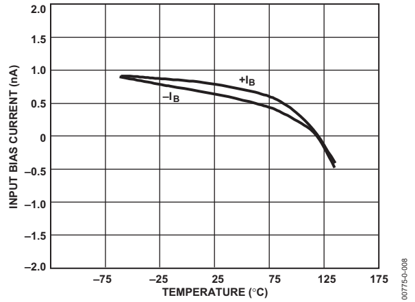
图8. 输入偏置电流与温度的关系
