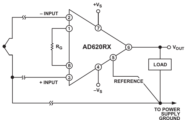
图48. 热电偶输入偏置电流的接地回路
