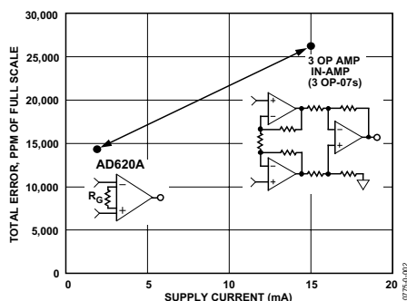
图2. 三运放分立仪表放大器设计与AD620RX比较
