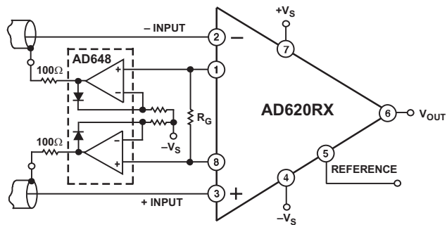
图44. 差分屏蔽驱动器
