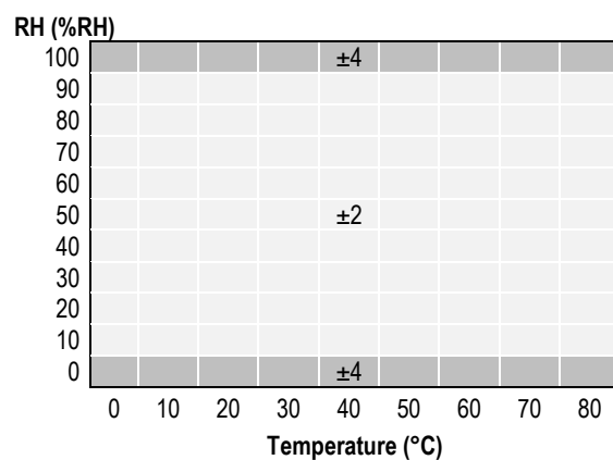
图3.1 不同温度条件下GXHT30的误差图
