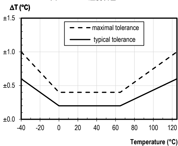
图 4 GXHT30 温度误差
