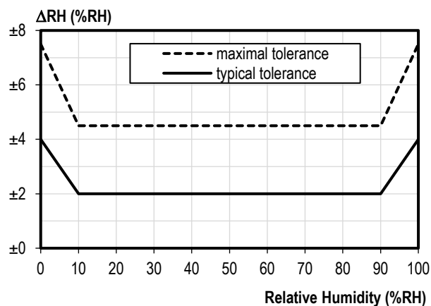
图 3 GXHT30 湿度误差@25° C
