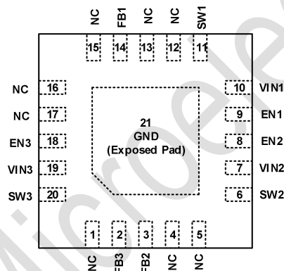
QFN3X3-20L
