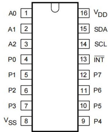
DIP-16/SOP-16/SOP-16W/QSOP-16/TSSOP-16
