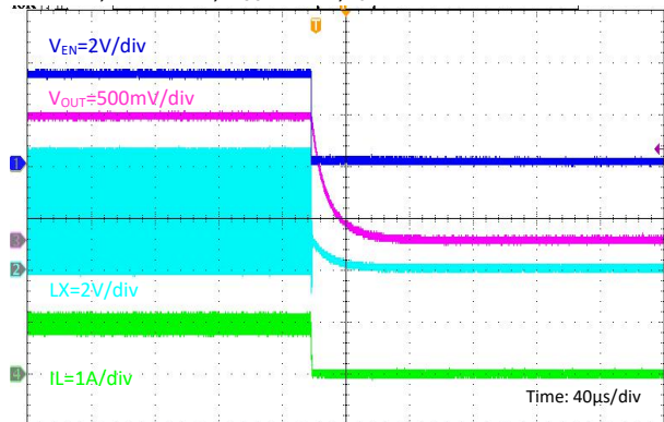
EN Enable Power Off
