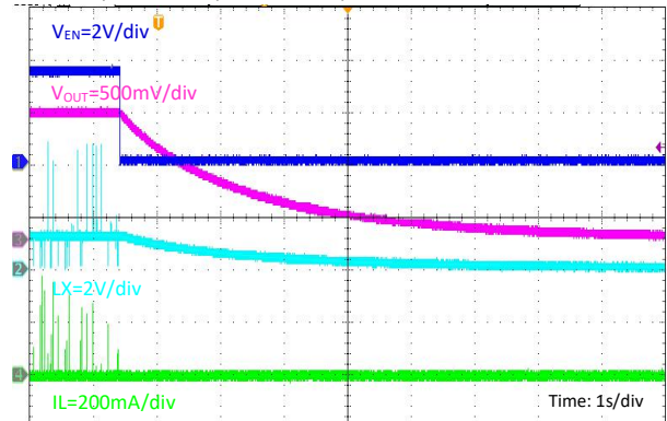
EN Disable Power Off
