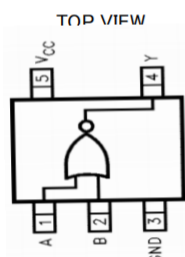
SOT23-5
