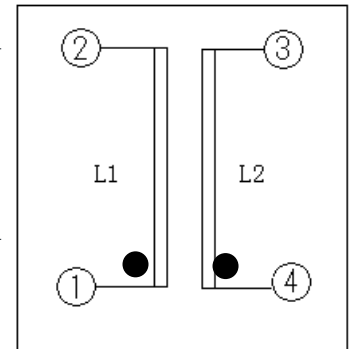
CONNECTION / 接线图
