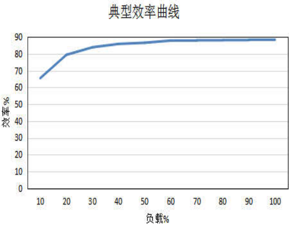
12V 输出典型效率曲线
