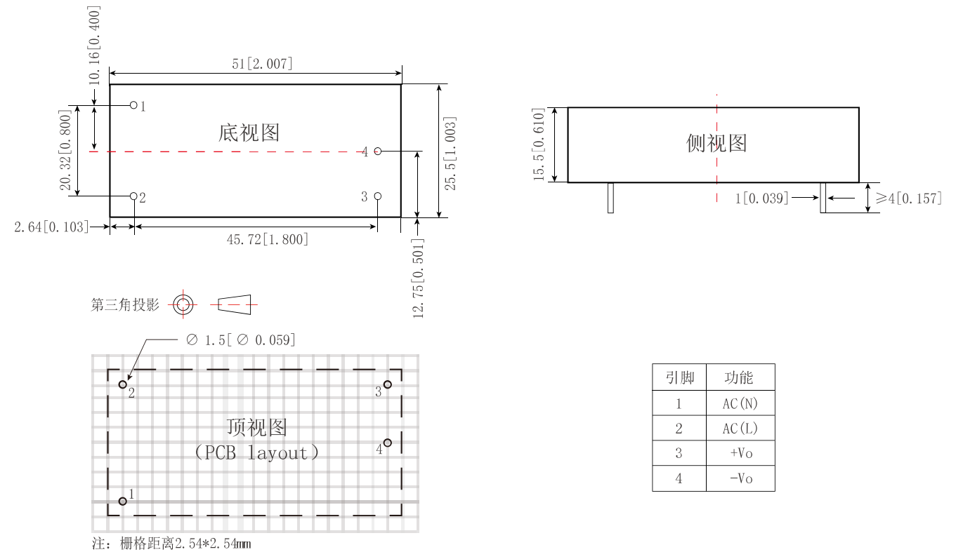
标准式封装
