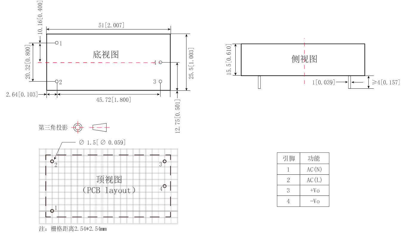
接线式 A/导轨式 D 封装
