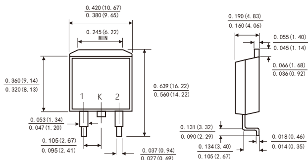
TO-263
