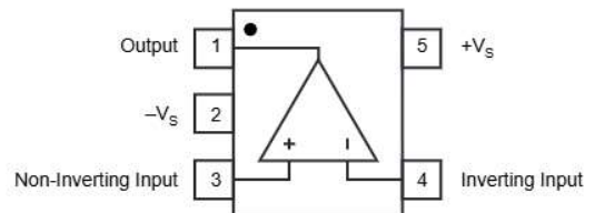
SOT23-5
