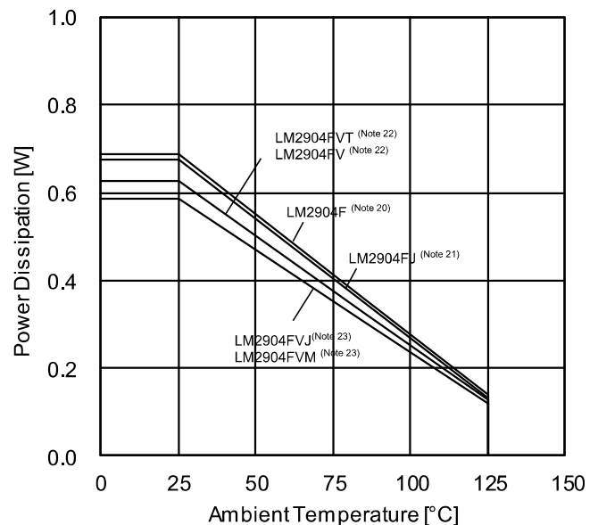
(d) LM2904xxx
