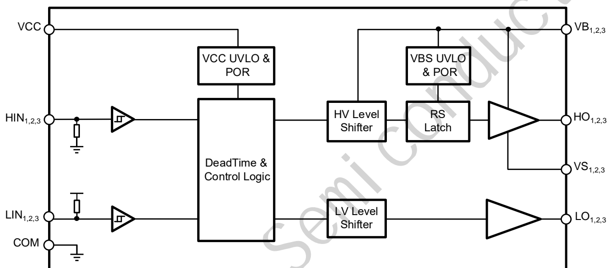
图 7-1 JSM2134功能框图
