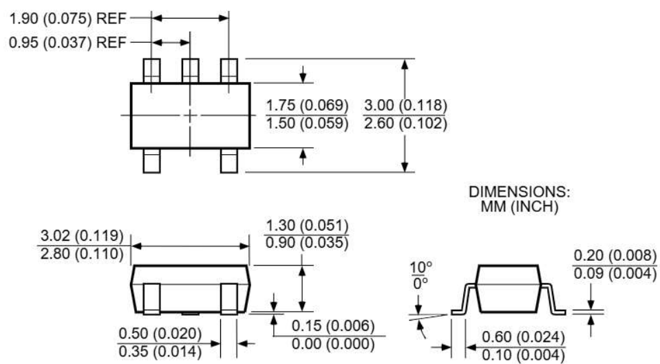
SOT-23-5 (M5)
