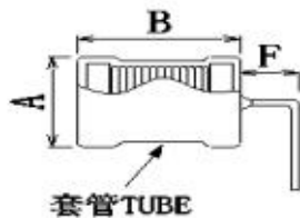
正视图 FRONT VIEW
