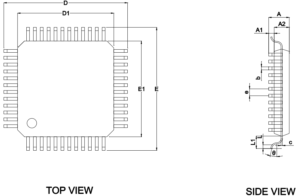
图 4-3 LKS32MC454CCT8 封装图示
