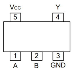
SOT23-5/ SOT353
