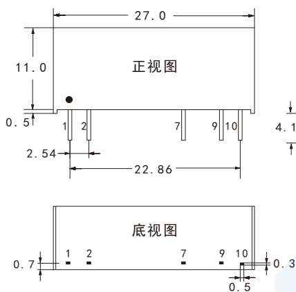
1) 外观尺寸
