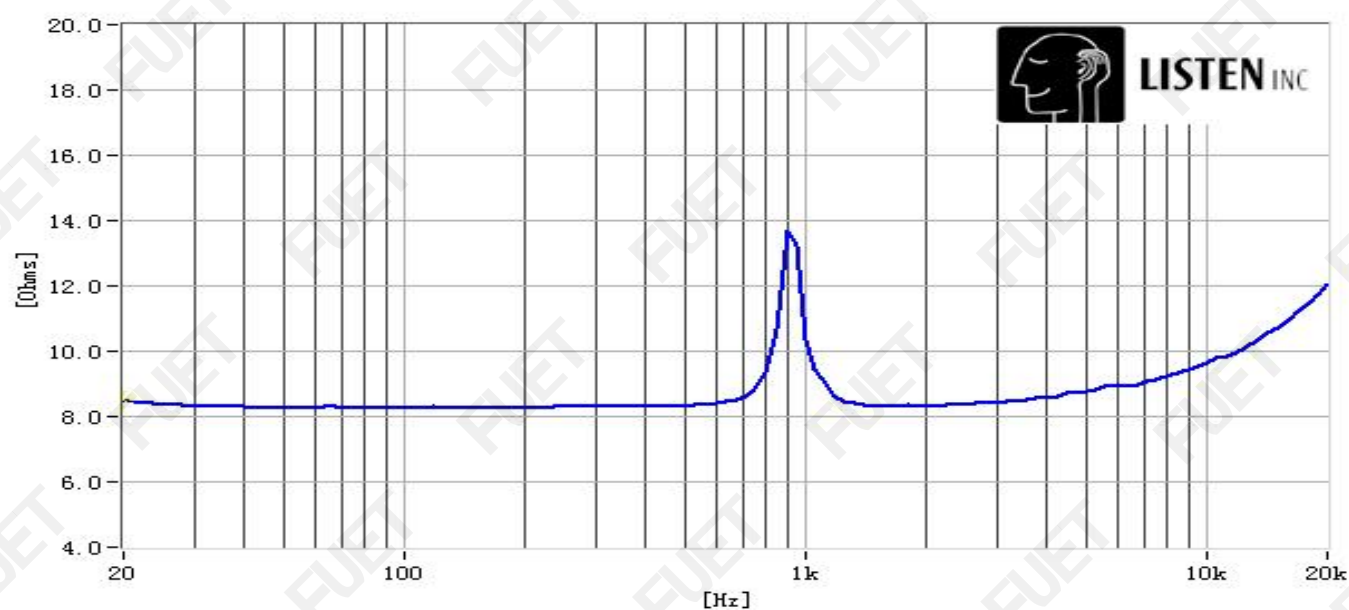
阻抗曲线
