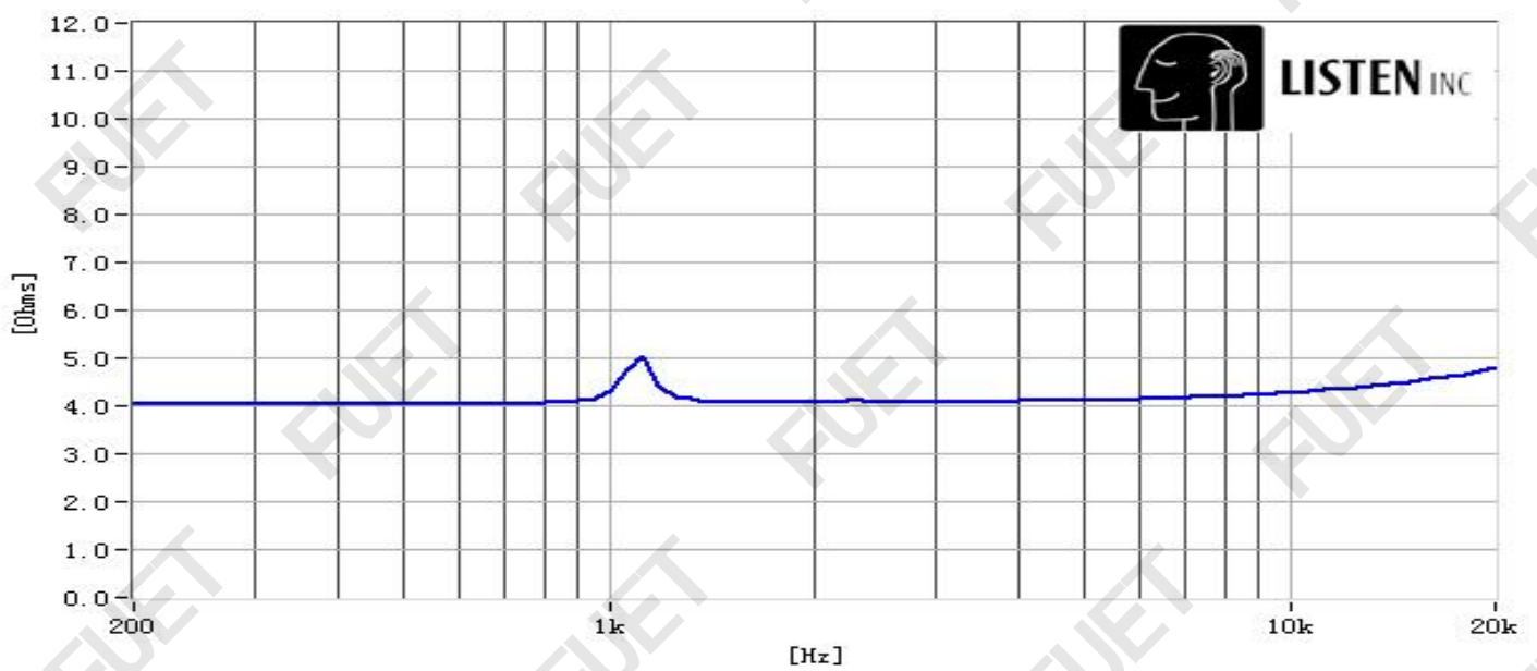
阻抗曲线
