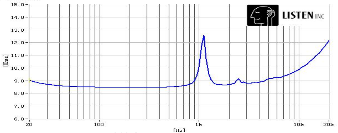
阻抗曲线
