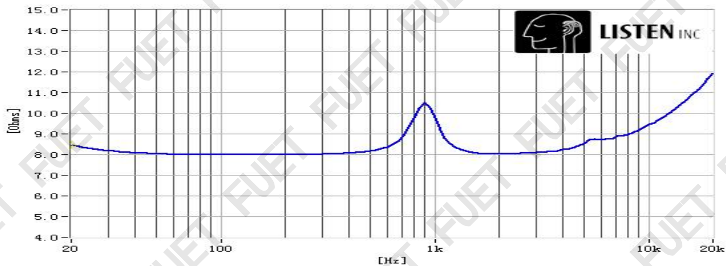
阻抗曲线
