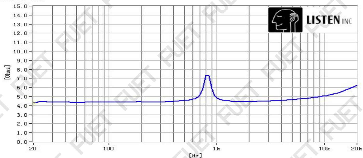
阻抗曲线
