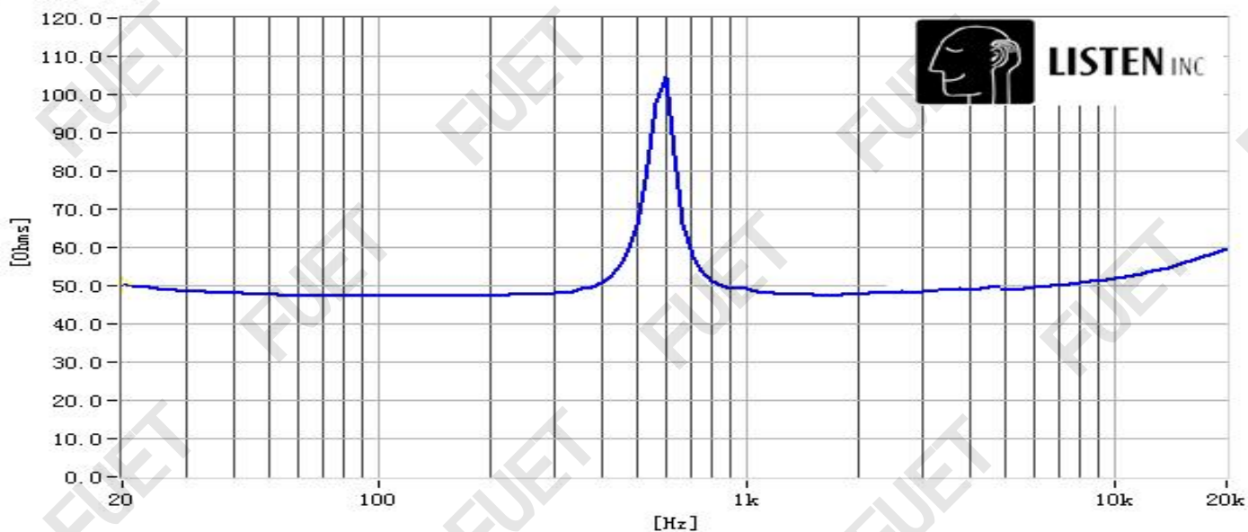
阻抗曲线
