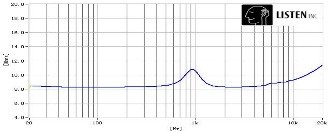
阻抗曲线
